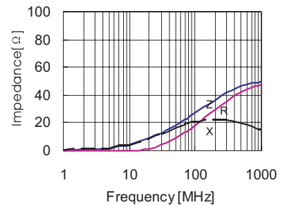
CBM201209U600T
