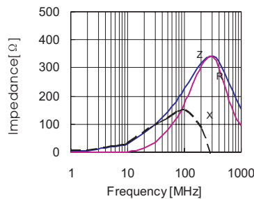
CBM201209U221T
